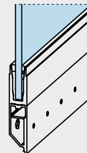
Basisprofil mit Unterbau für erhöhten Fußbodenaufbau Profilé de base avec socle pour montage surélevé Basisprofiel met onderconstructie voor verhoogde vloerconstructie
