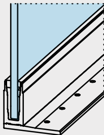
Basisprofil mit Unterbau zur Kantenmontage Profilé de base avec socle pour montage déporté Basisprofiel met onderconstructie voor randmontage
