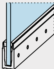
Basisprofil Profilé de base Basisprofiel
