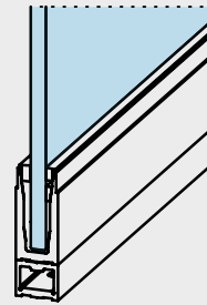
Basisprofil mit Unterbau für erhöhten Fußbodenaufbau Profilé de base avec socle pour montage surélevé Basisprofiel met onderconstructie voor verhoogde vloerconstructie
