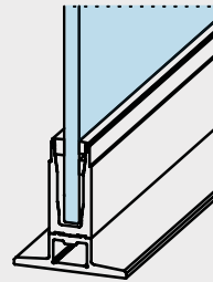
Basisprofil mit Unterbau mit breitem Fußpunkt für erhöhten Fußbodenaufbau Profilé de base avec socle pour montage déporté et surélevé Basisprofiel met onderconstructie voor randmontage voor verhoogde vloerconstructie
