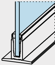
Basisprofil mit Unterbau mit breitem Fußpunkt Profilé de base avec socle élargi Basisprofiel met onderconstructie met brede voetplaat
