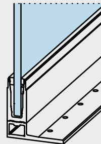
Basisprofil mit Unterbau zur Kantenmontage für erhöhten Fußbodenaufbau Profilé de base avec socle élargi pour montage surélevé Basisprofiel met onderconstructie met brede voetplaat voor verhoogde vloerconstructie
